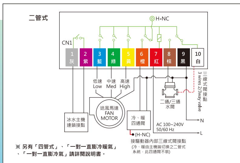
二管式 系統配線圖
